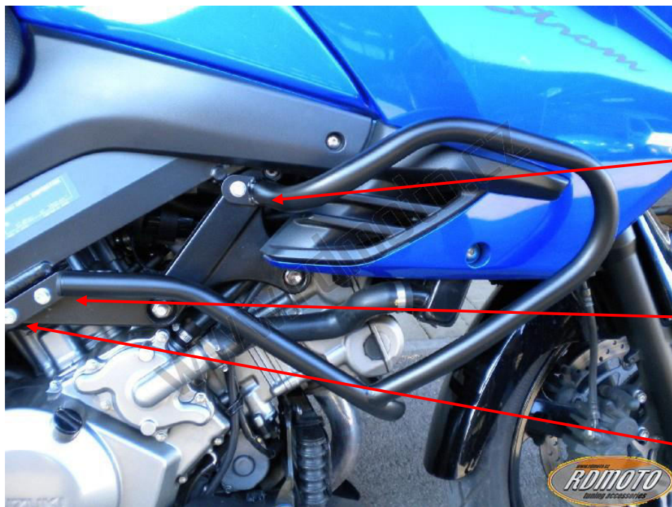
šroub M8x50mm k uchycení do rámu + duralový váleček 16mm + podložka pérová + krytka na hlavu šroubu
