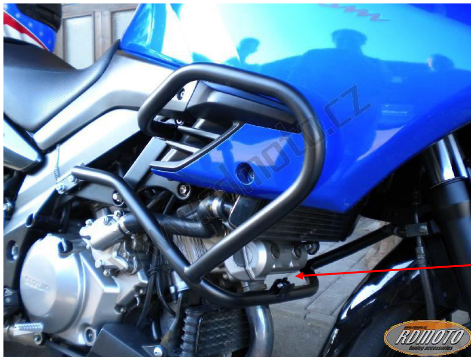
šroub M8x30mm pro spojení rámu
